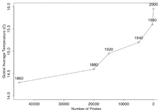
图 1: 全球平均温度与海盗活动, 源于 Henderson, 2006
